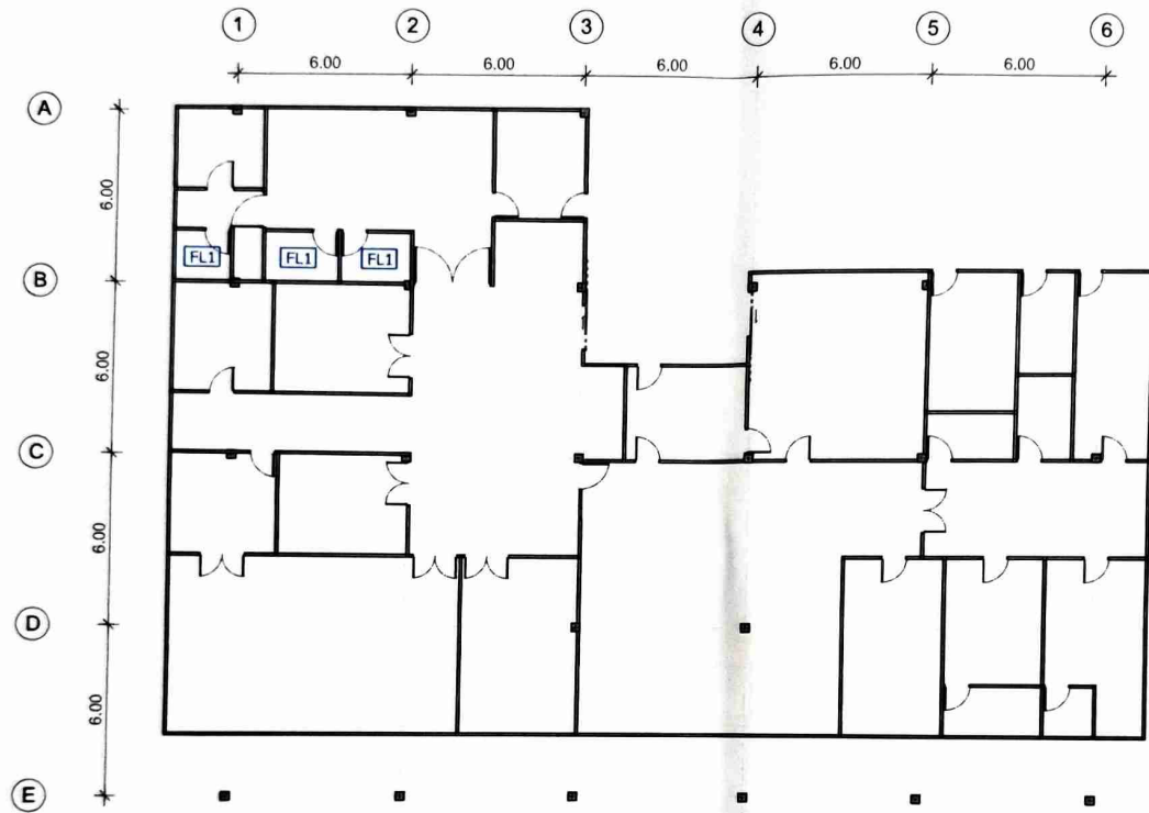
ผังแสดงงานพื้น SCALE 1 : 200
