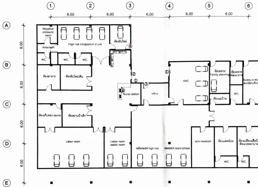
ผังงานประตูและหน้าต่าง SCALE 1 : 200
