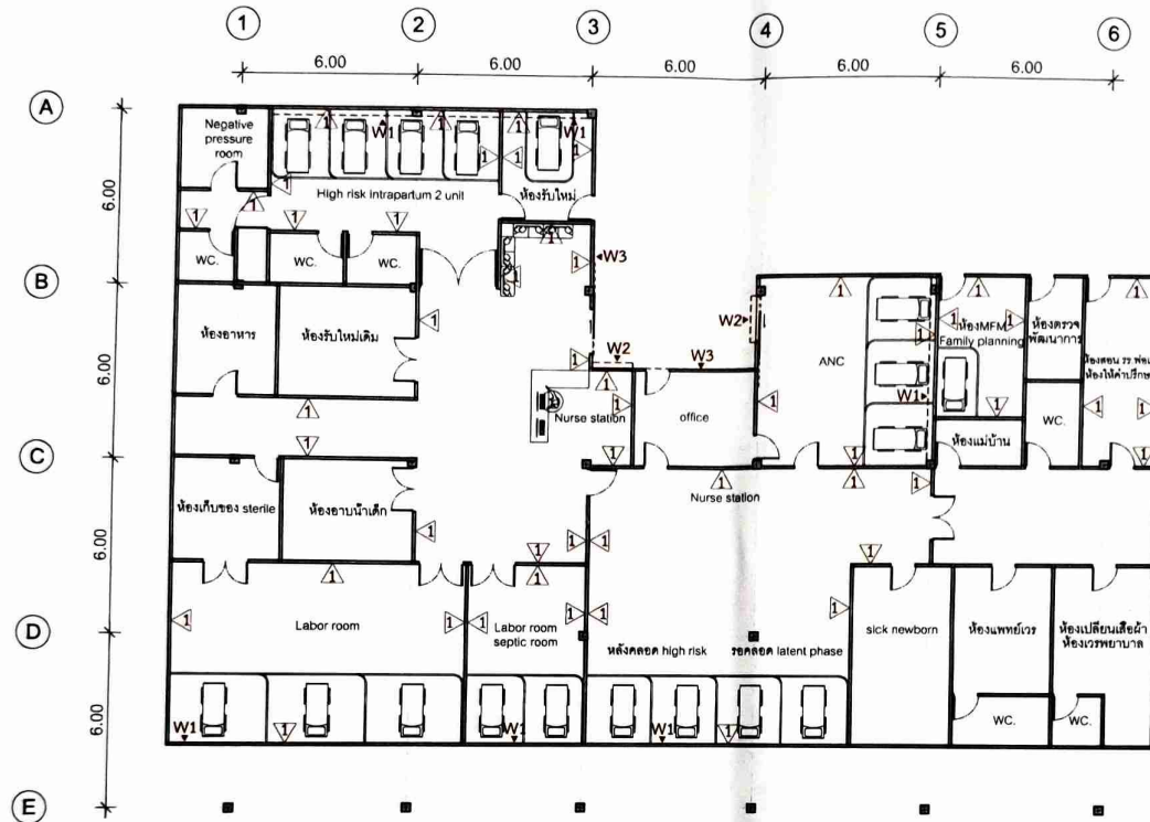
ผังงานแสดงงานผนังและทาสี SCALE 1 : 200
